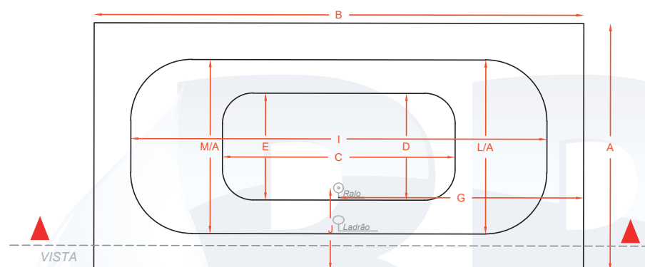
Planta baixa
