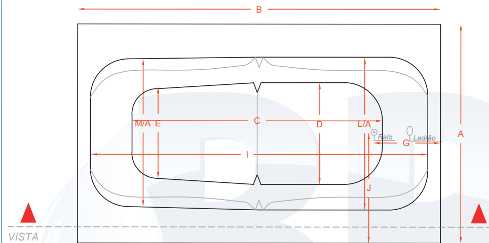
Planta baixa
