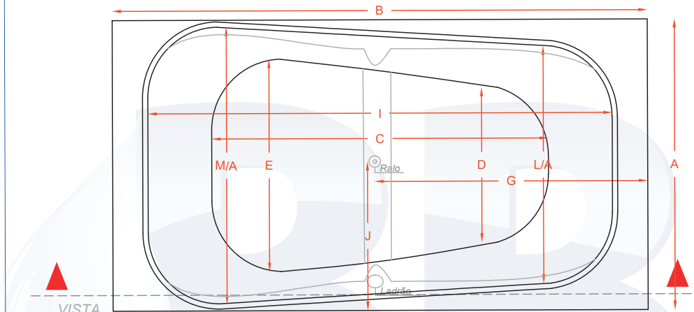
PLANTA BAIXA
