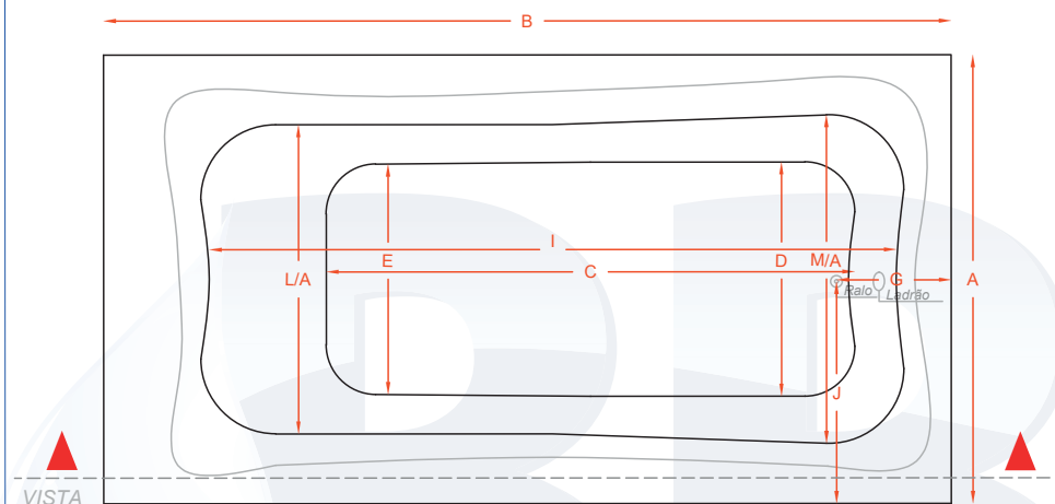
PLANTA BAIXA
