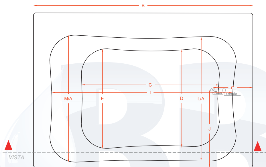
Planta baixa
