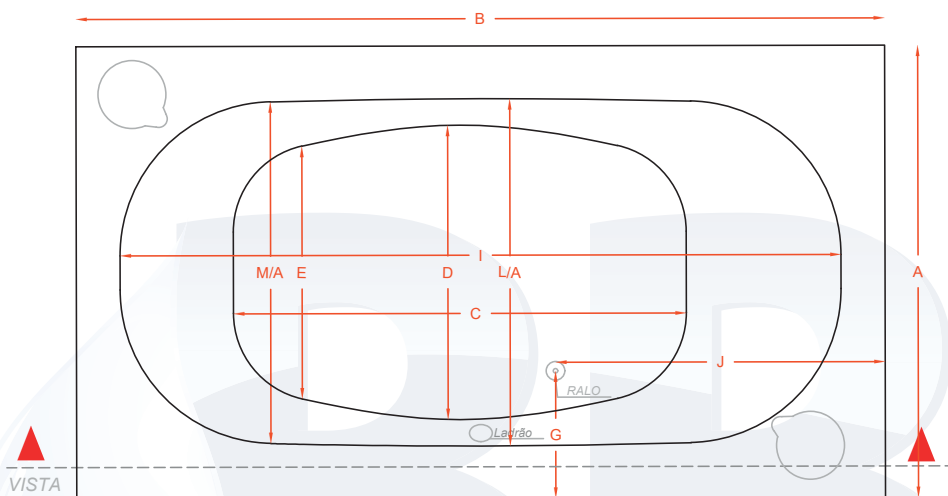
PLANTA BAIXA
