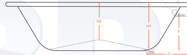
VISTA LATERAL
